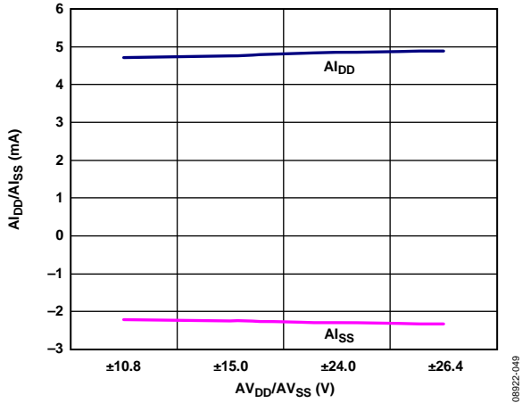
Figure 47. I_{DD}/I_{SS} vs. V_{DD}/V_{SS} , V_{OUT} = 0 V
